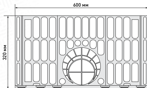
вид сбоку (с поддоном)
