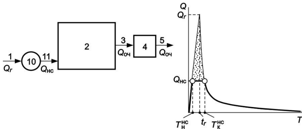
Рис. 1. Схема перекачки полного объема незарегулированного дождевого стока 1 – 5 – см. рис. 1, п. 7.2.4; 10 – насосная станция; 11 – напорный трубопровод перекачки стока в аккумулирующий резервуар; □ часть объема дождя, поступающего в аккумулирующий резервуар для последующей очистки; ▨ рабочий объем резервуара насосной станции
