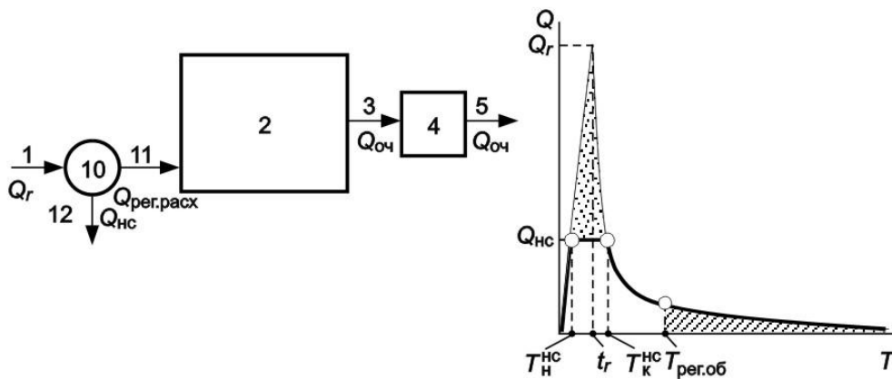
Рис. 2. Схема перекачки избыточной части зарегулированного по объему дождевого стока 1 – 5, 10, 11 – см. рис. 1; 12 – напорный трубопровод перекачки избыточного стока; □ часть объема дождя, поступающего в аккумулирующий резервуар для последующей очистки; ▨ часть объема дождя, отводимого в водный объект без очистки; ▩ рабочий объем резервуара насосной станции
